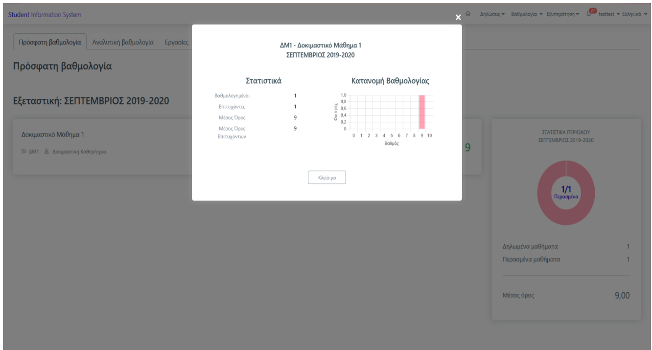
Εικ. 8.2: Στατιστικά
